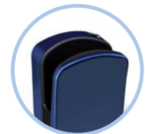
Deep Blue
